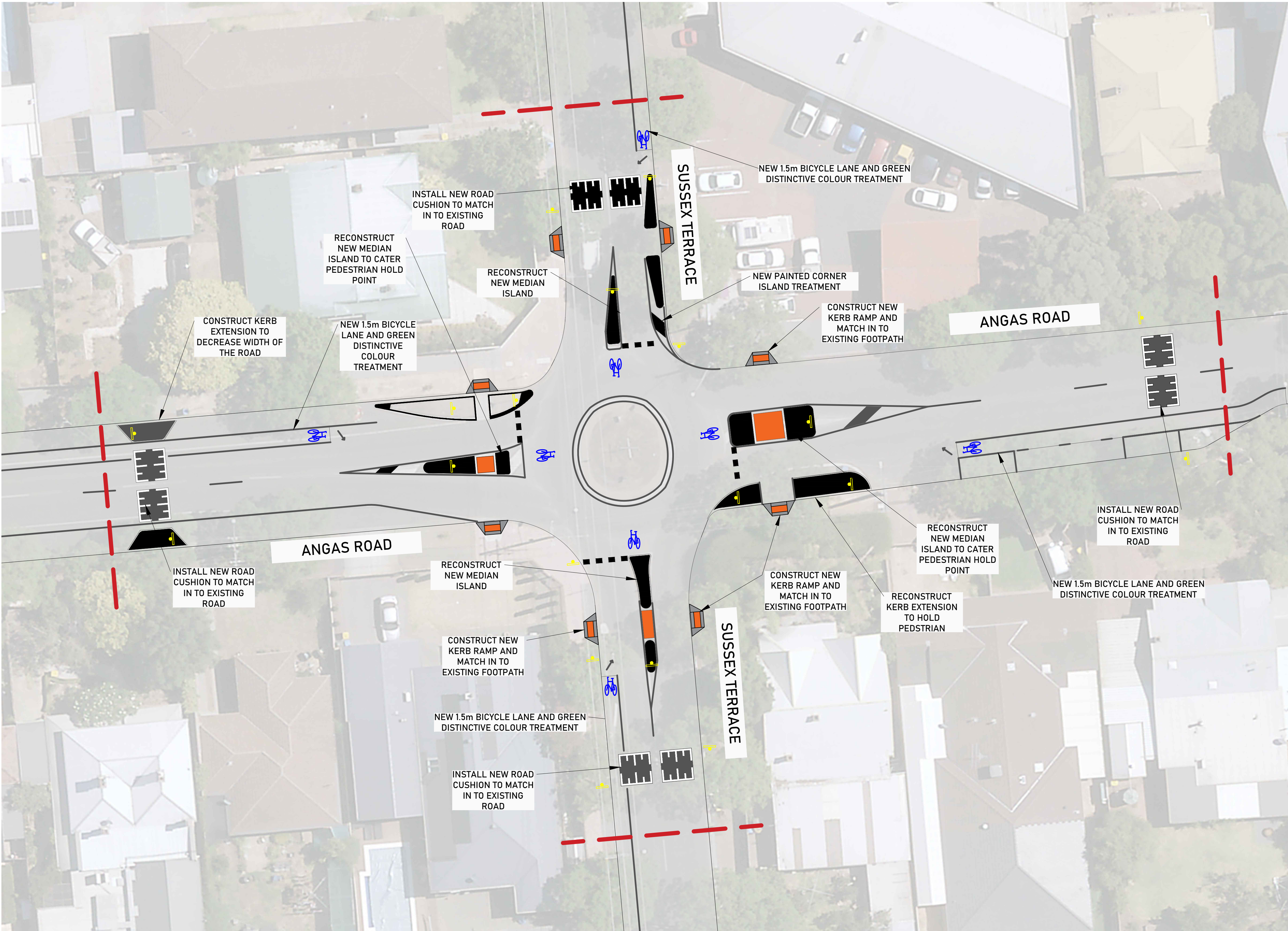
ANGAS RD - SUSSEX TCE ROUNDABOUT SCALE: 1:200 @ A1
